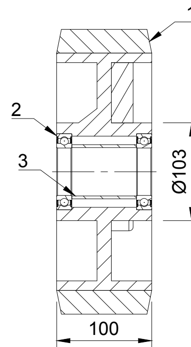
A-A (1:4)
