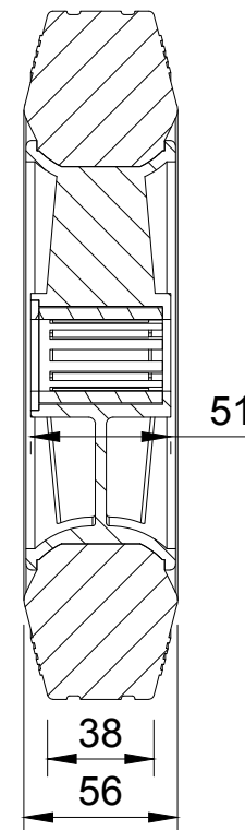
A-A (1:3)
