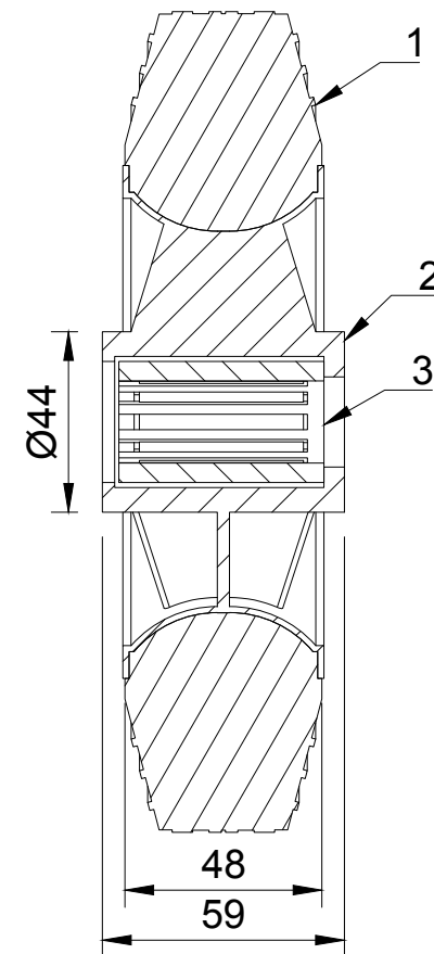
A-A (1:2)
