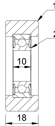
A-A (1:1)
