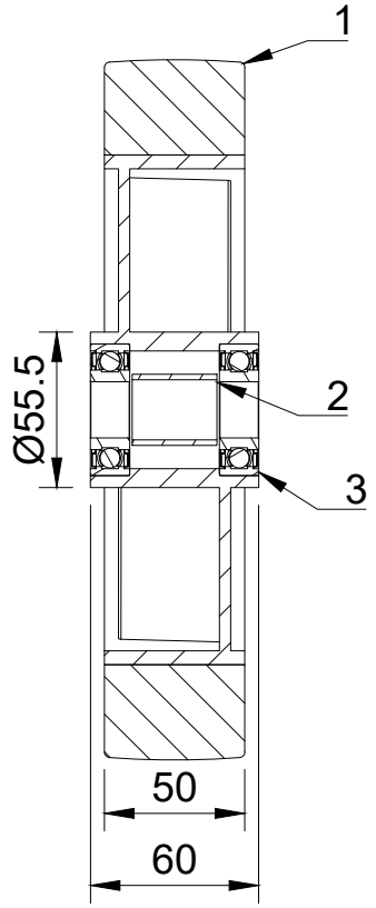
A-A (1:3)
