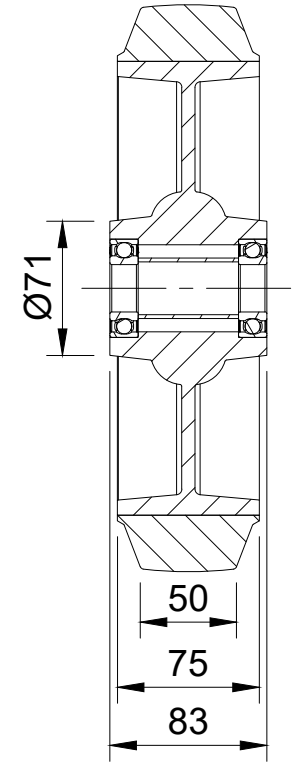
A-A (1:4)
