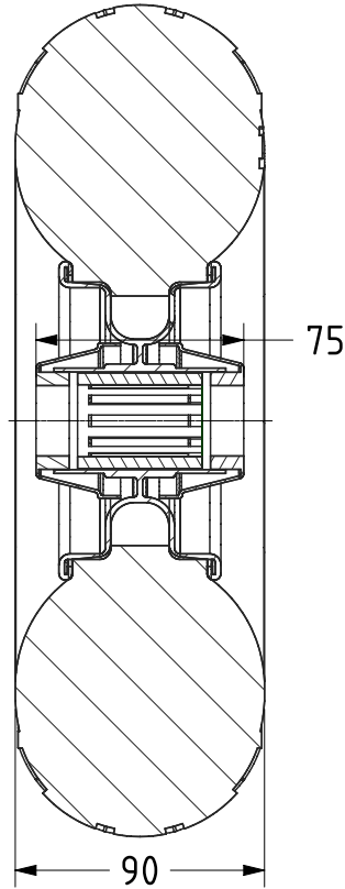
SECTION A-A
