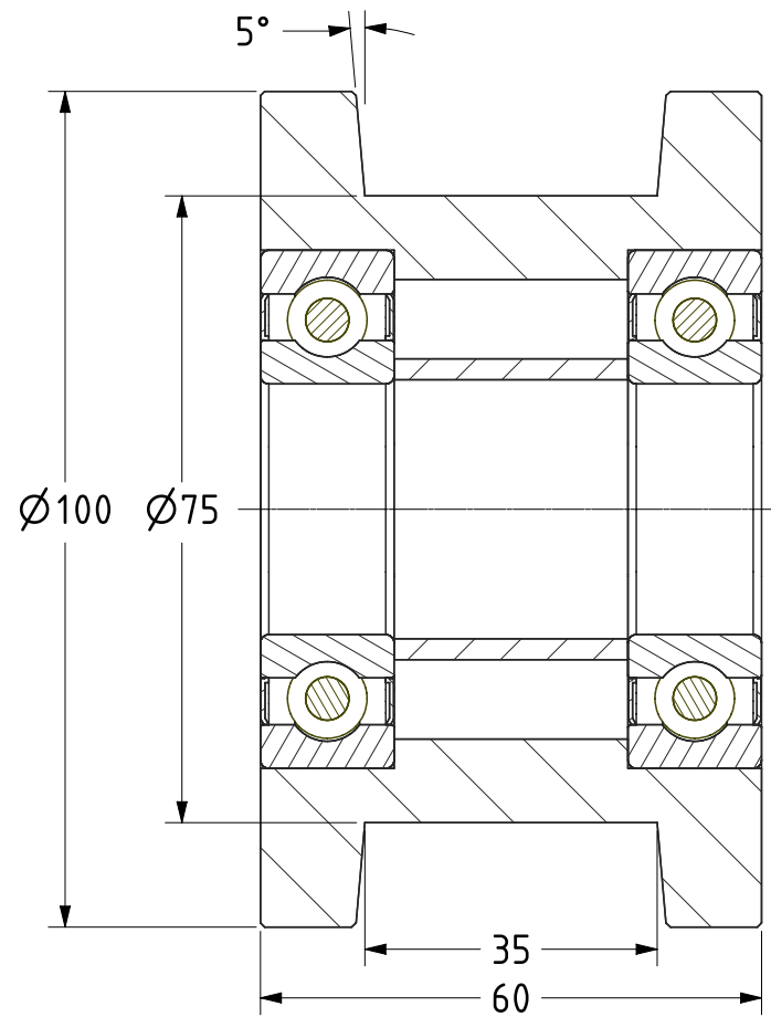
SECTION A-A
