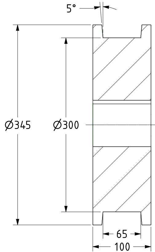
SECTION A-A
