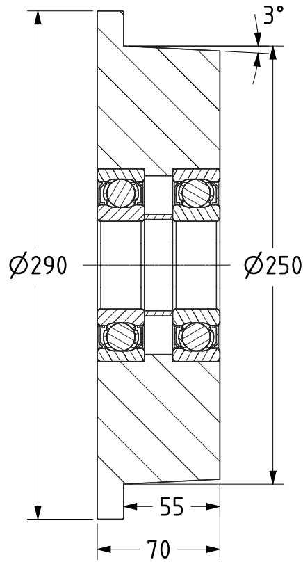
SECTION A-A
