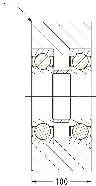
SECTION A-A
