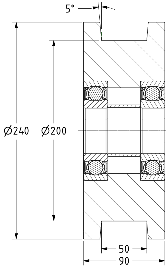
SECTION A-A
