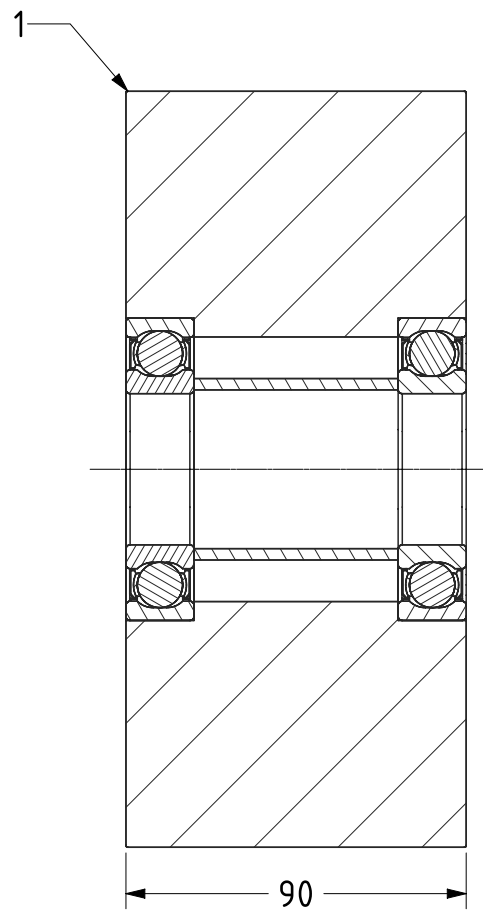
SECTION A-A
