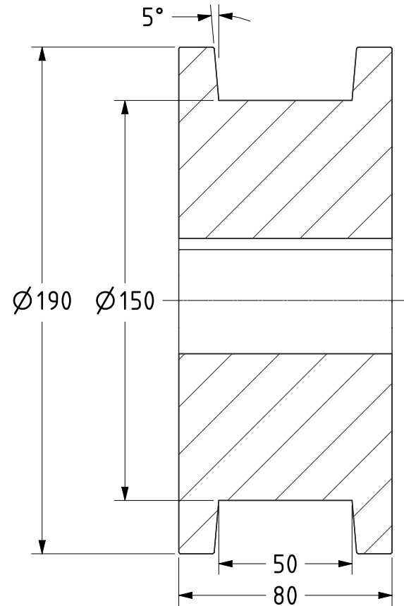
SECTION A-A
