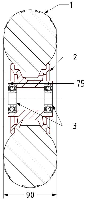
SECTION A-A
