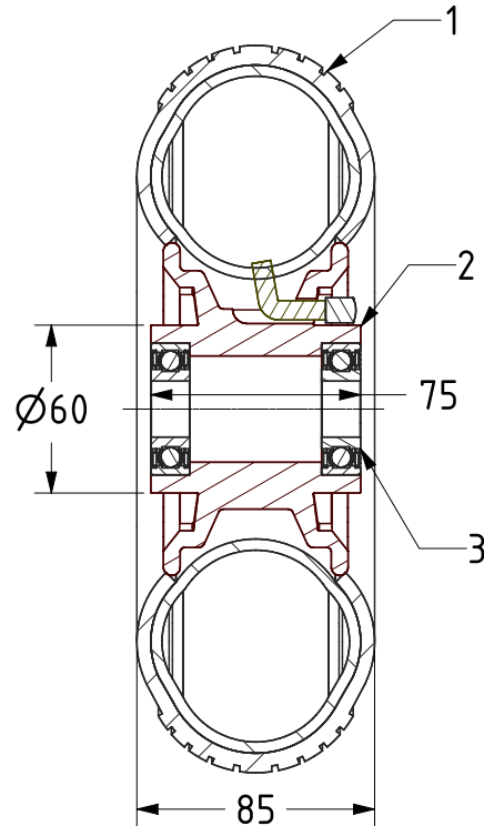
SECTION A-A
