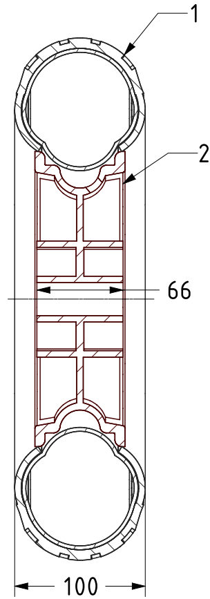
SECTION A-A
