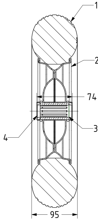
SECTION A-A
