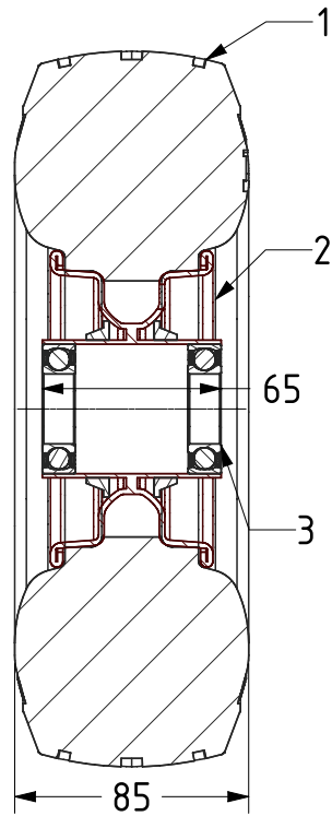
SECTION A-A
