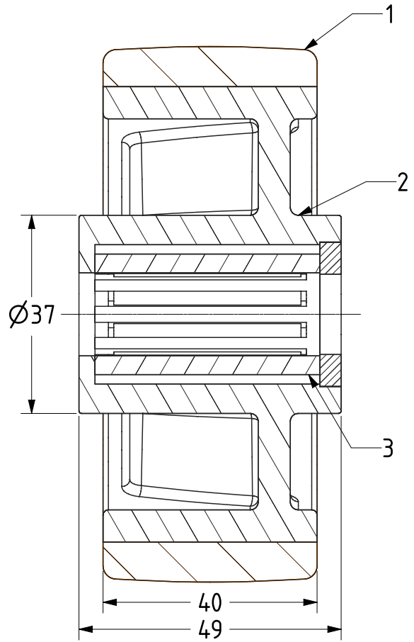
SECTION A-A
