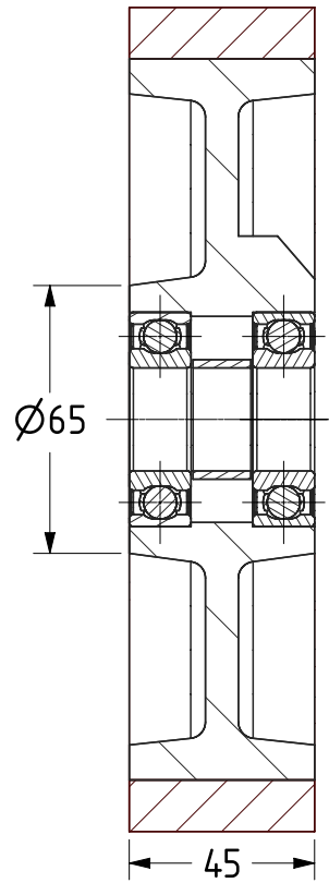
SECTION A-A
