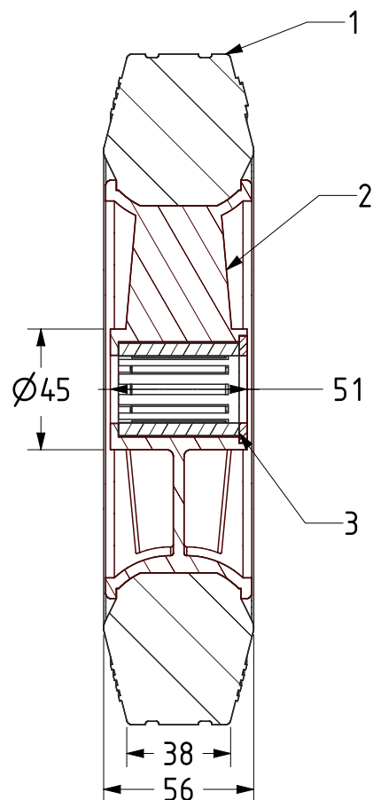
SECTION A-A
