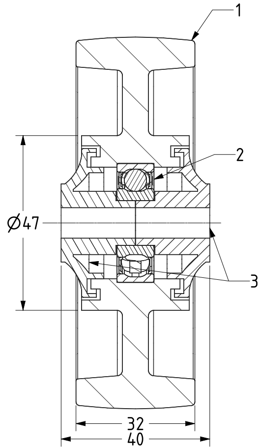
SECTION A-A
