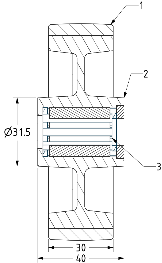
SECTION A-A
