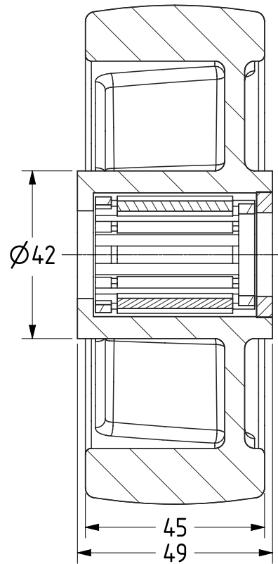
SECTION A-A
