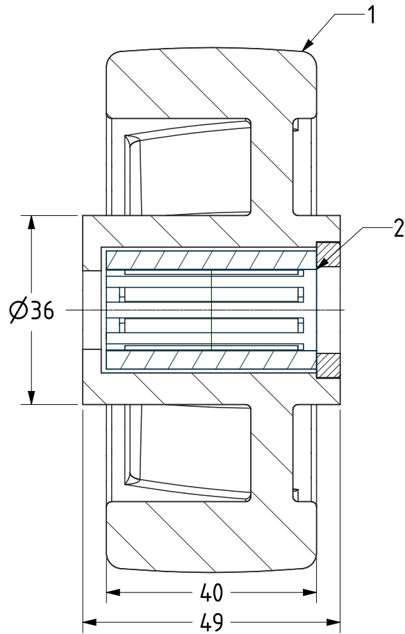
SECTION A-A
