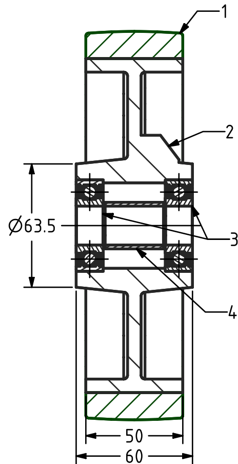
SECTION A-A
