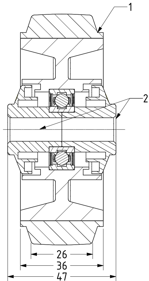
SECTION A-A
