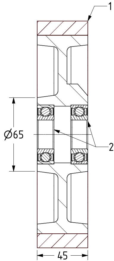
SECTION A-A
