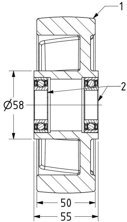
SECTION A-A
