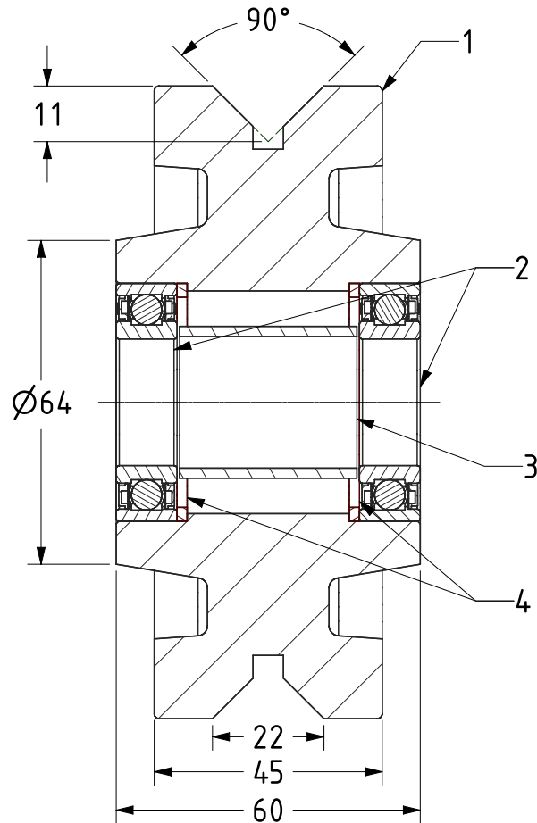
SECTION A-A
