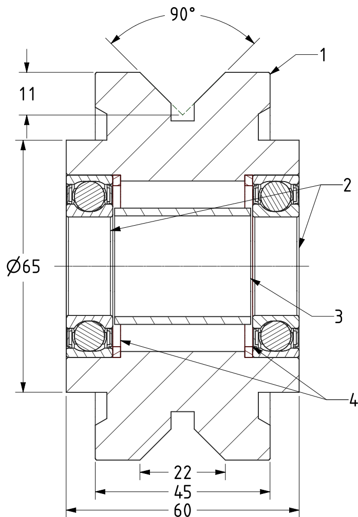
SECTION A-A
