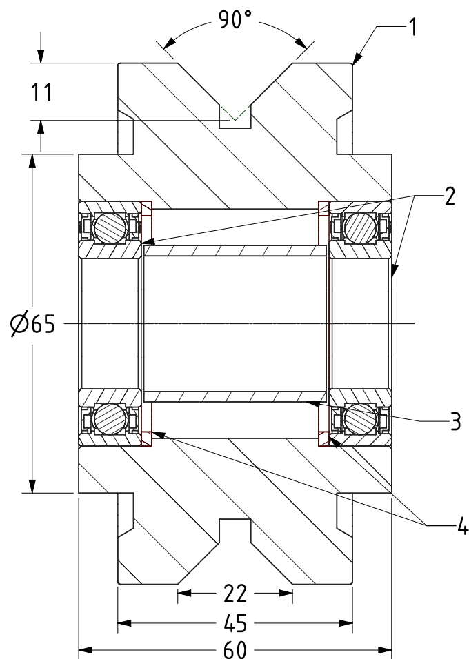
SECTION A-A
