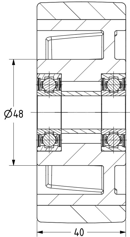
SECTION A-A
