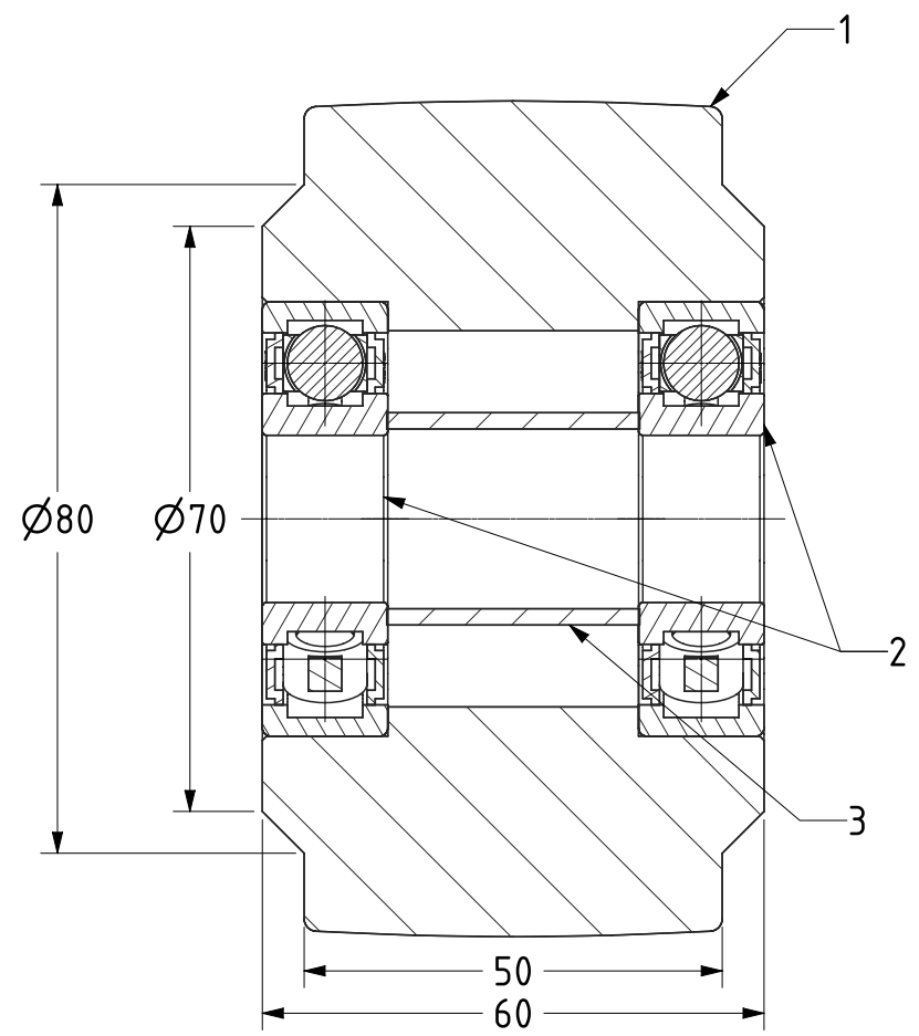
SECTION A-A
