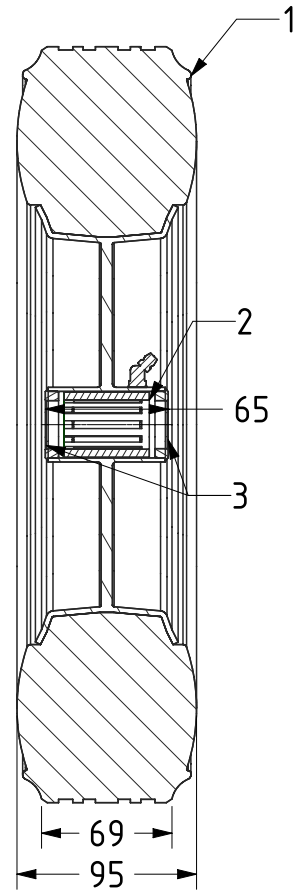
SECTION A-A
