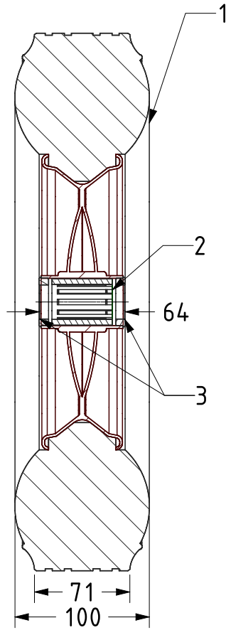
SECTION A-A
