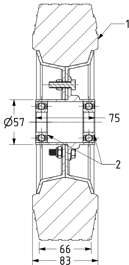
SECTION A-A
