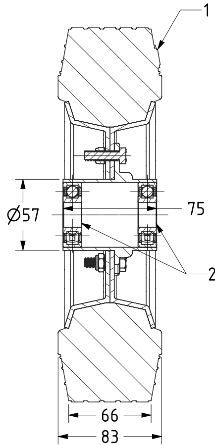
SECTION A-A
