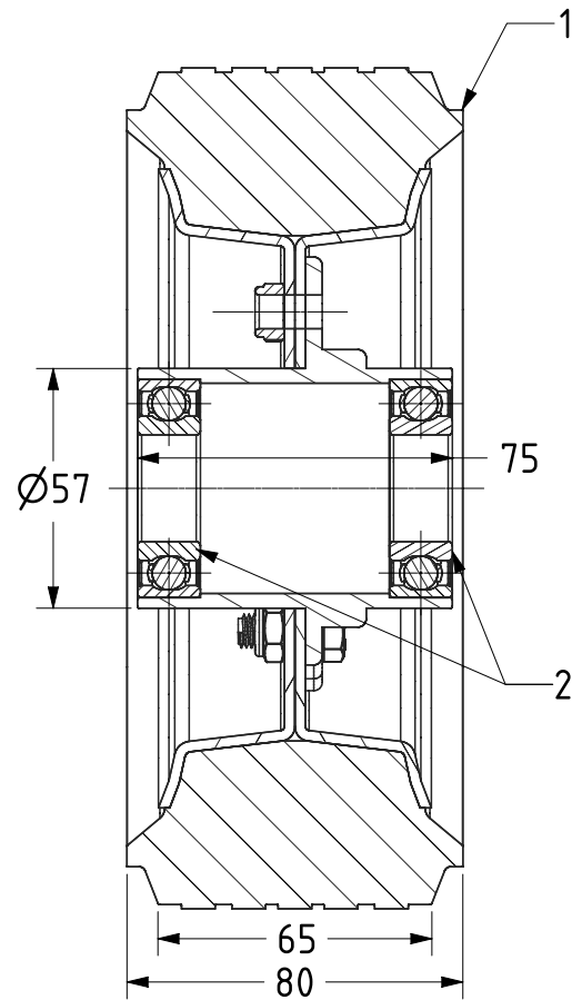
SECTION A-A
