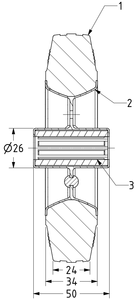
SECTION A-A
