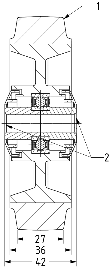
SECTION A-A
