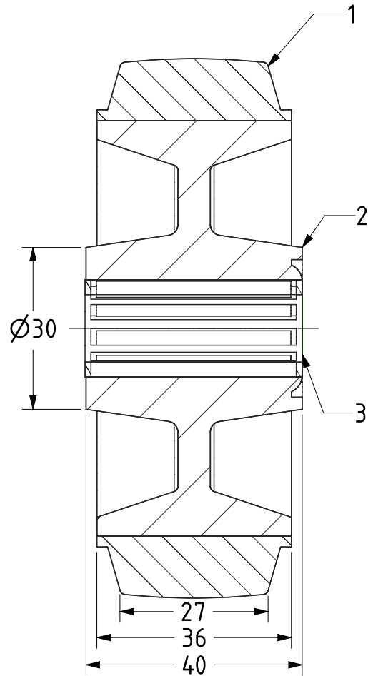
SECTION A-A
