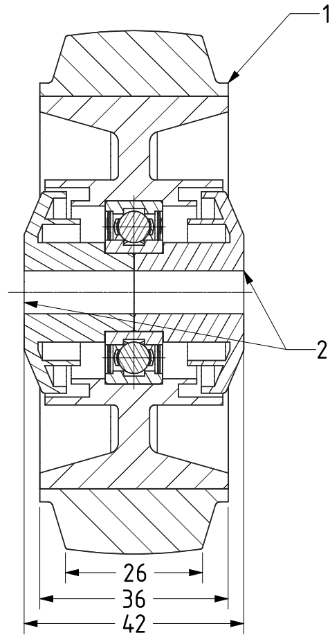
SECTION A-A
