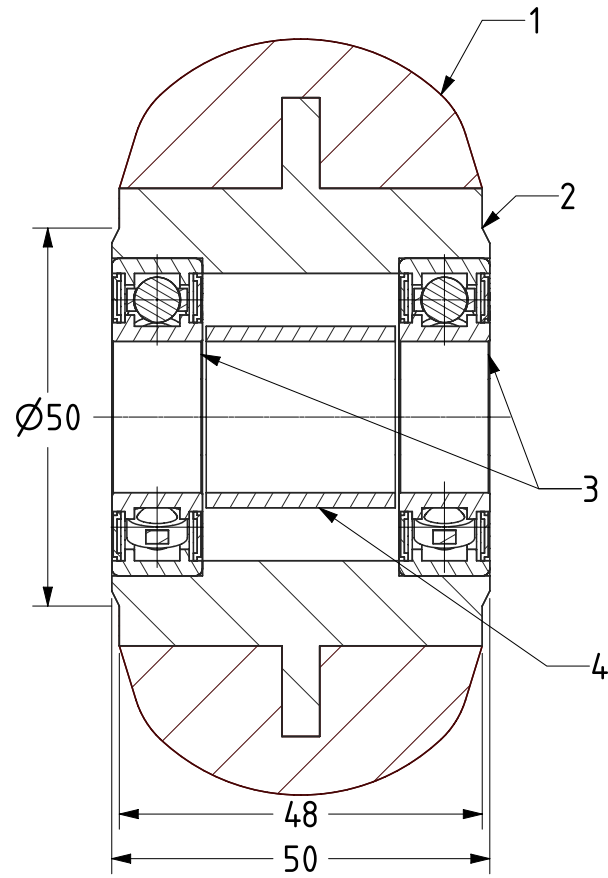
SECTION A-A
