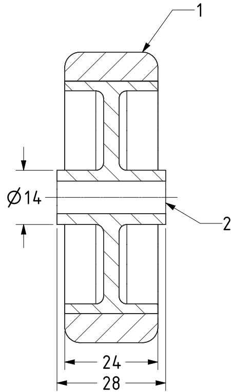
SECTION A-A
