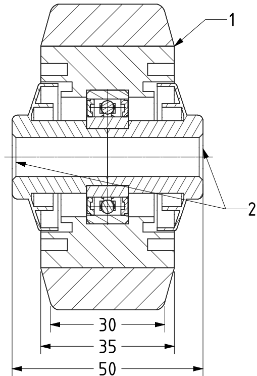
SECTION A-A
