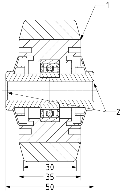
SECTION A-A
