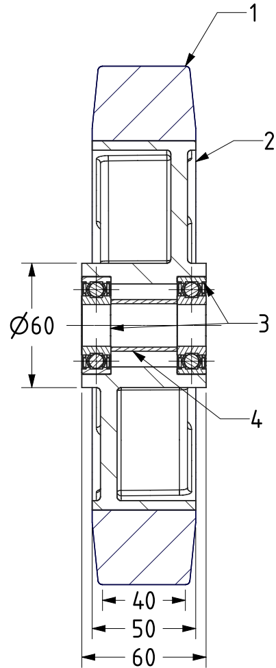
SECTION A-A
