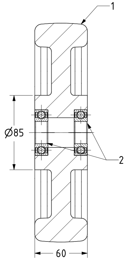
SECTION A-A
